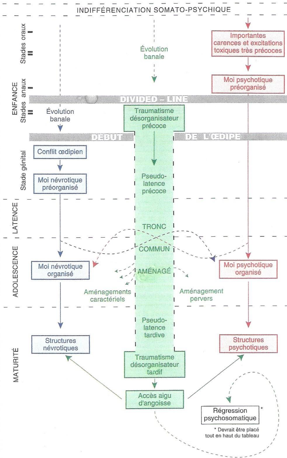
FIGURE 8 : Synthèse de la genèse et de l'évolution des lignées structurelles.
